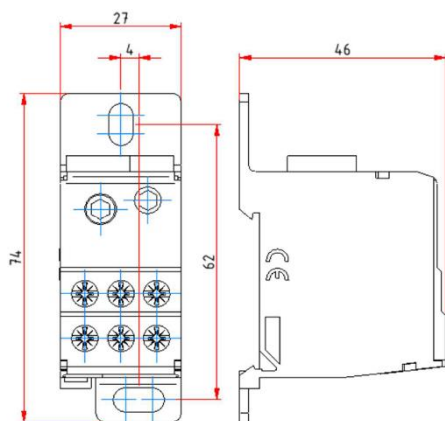
Dimensional Drawing | Plan d'encombrement
